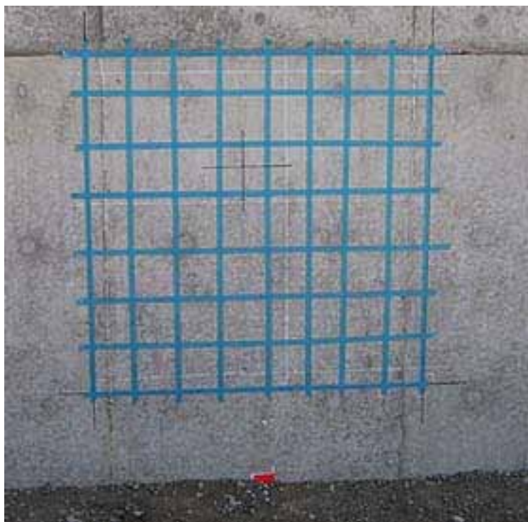
山側柱面配筋状況写真
