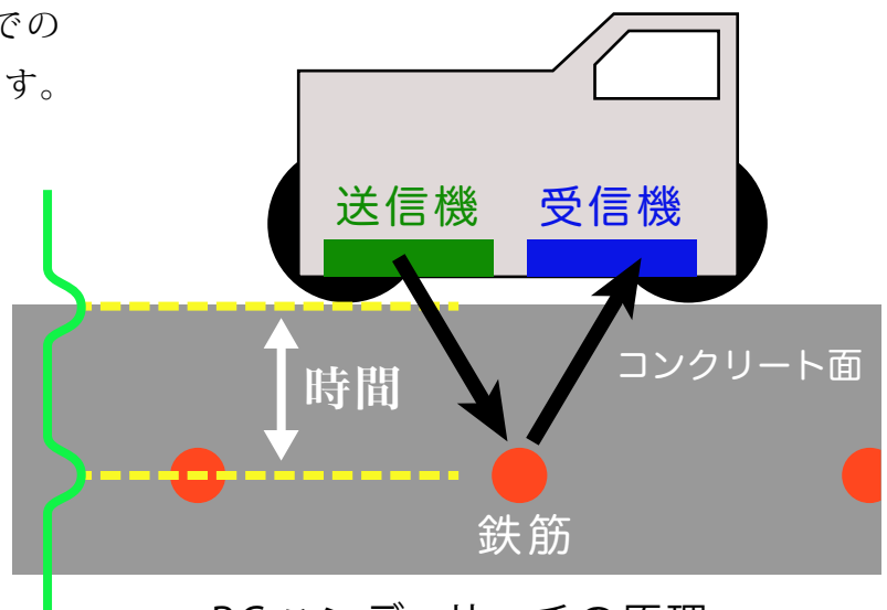
RCハンディサーチの原理
